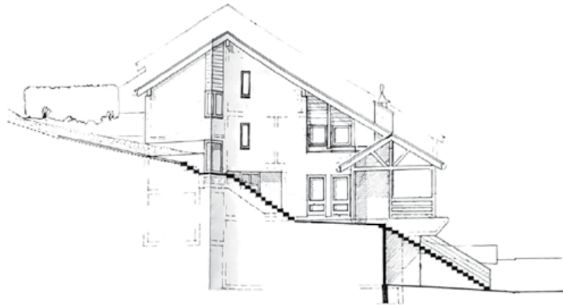
Nordfassade
